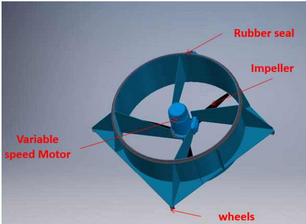
Motor fan
